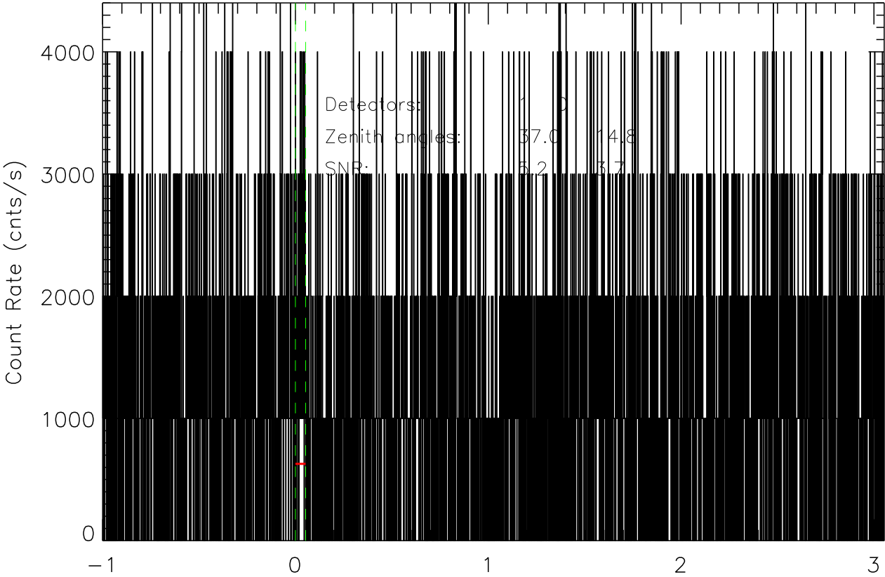
SGR J1550-5418 Burst ID:254278482
